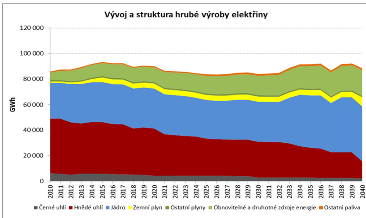
Obrázek 37: Vývoj a struktura hrubé výroby elektřiny v rámci Optimalizovaného scénáře SEK
