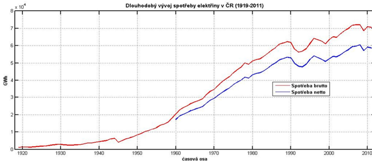
Obrázek 36: Dlouhodobý vývoj spotřeby elektřiny v ČR (1919-2011)
